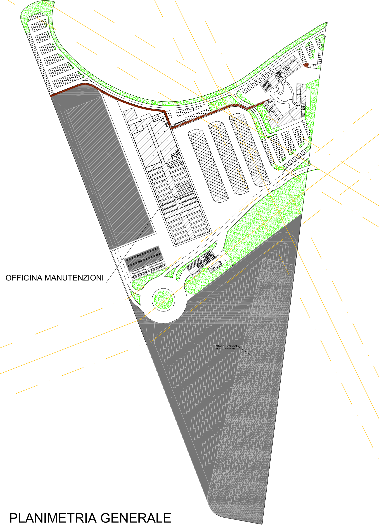
PLANIMETRIA GENERALE
